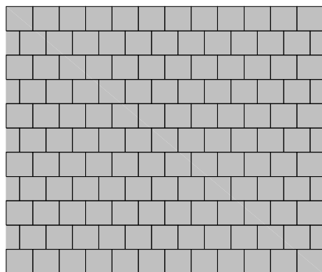
Bedarf 14 x 14 cm ca. 50 St/m 2
