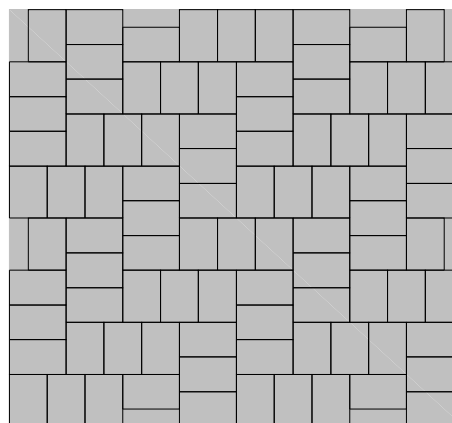
Bedarf 14 x 21 cm ca. 33 St/m 2
