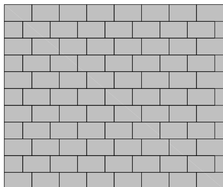
Bedarf 14 x 21 cm ca. 33 St/m 2 Randabschluß 14 x 14 cm
